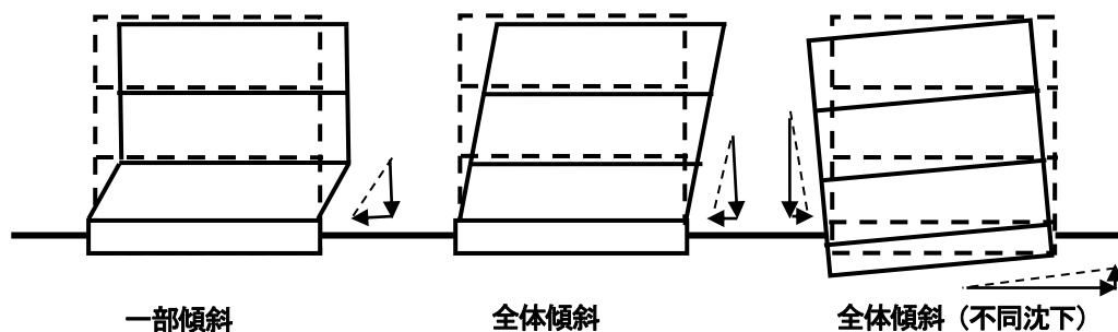
図3-4 鉄骨造建築物の傾斜
