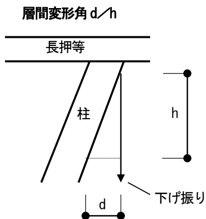
図2-1 傾斜の測定
