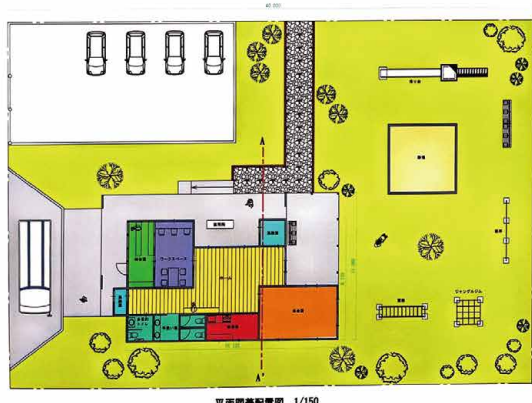
平面図案配置図 1/150
